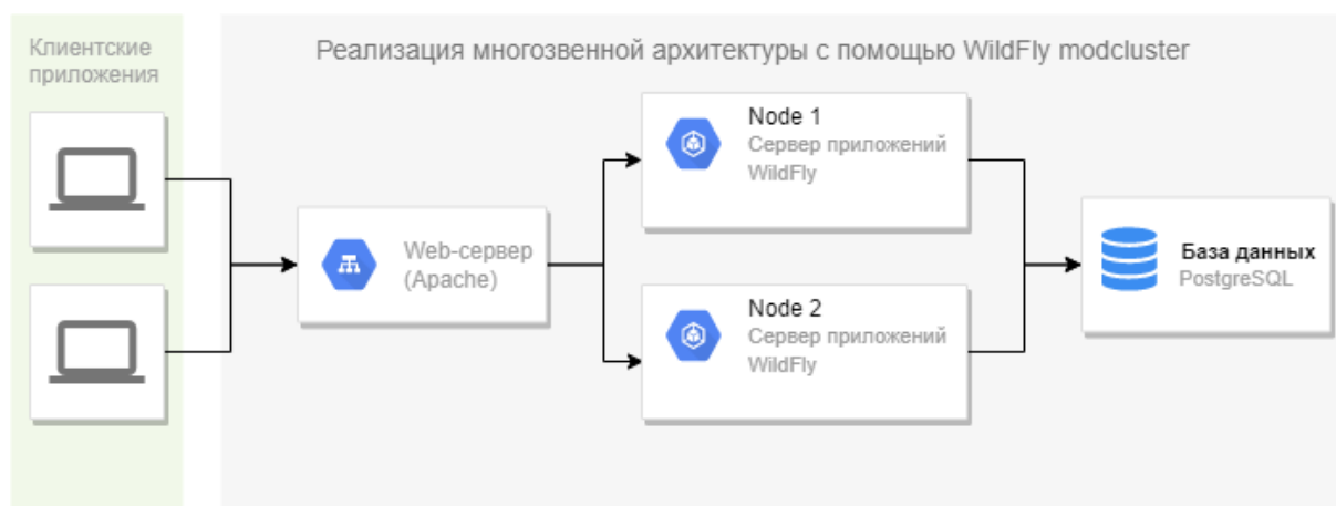
Рисунок 1 — Реализация многозвенной архитектуры ИАС ОПОВС/ПОРДТС
